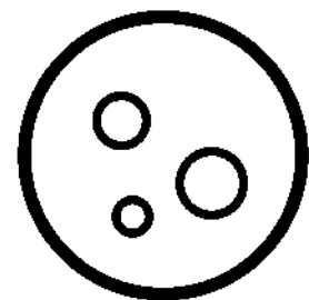
Titania
