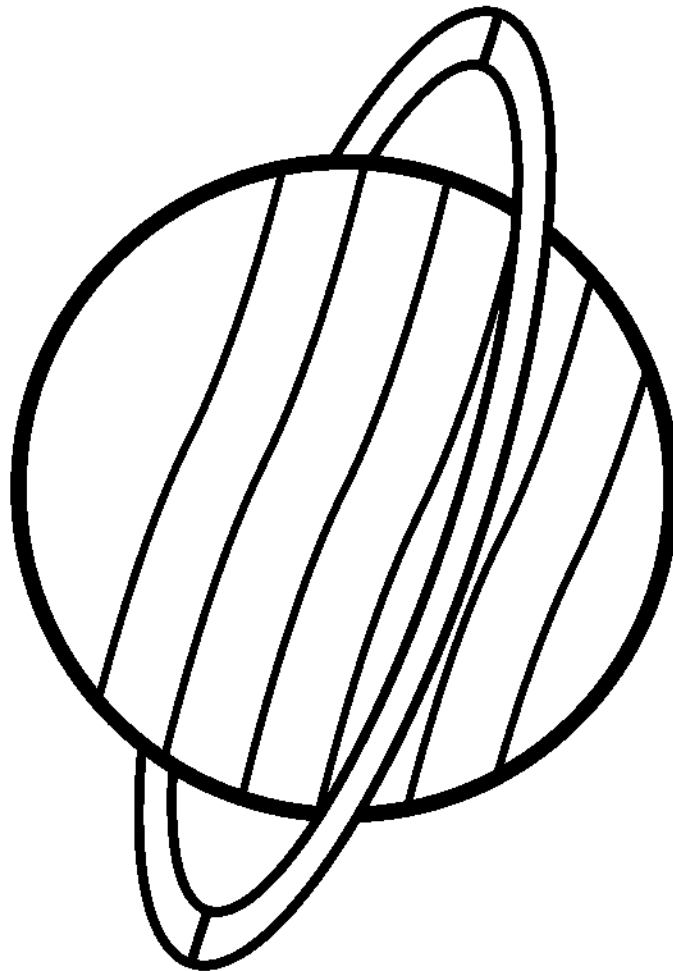
URANUS
