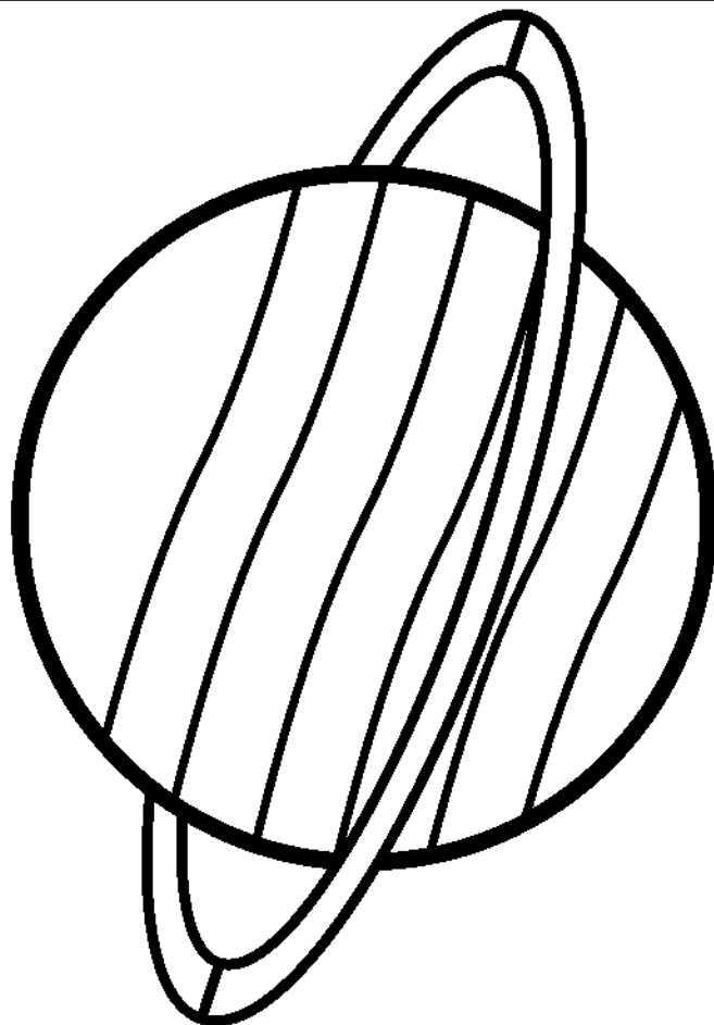
URANUS
