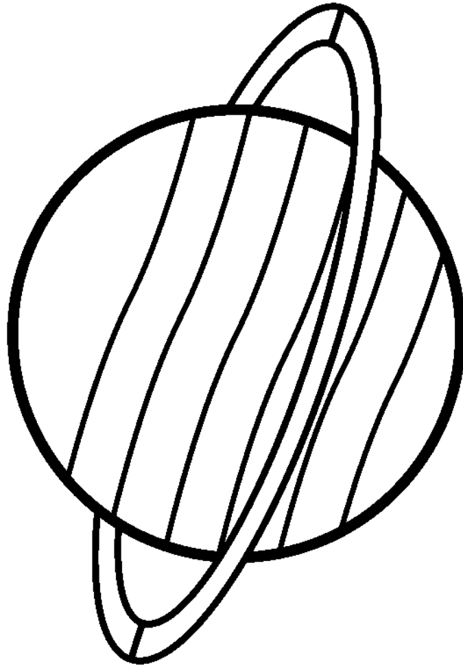
URANUS
