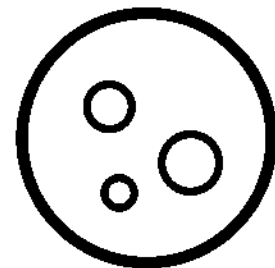
Mimas
