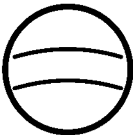
Titan
