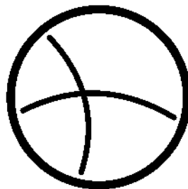
Enceladus
