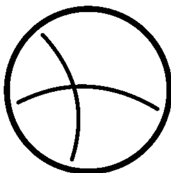
Enceladus
