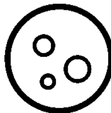
Ganymede
