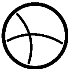
Europa
