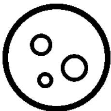
Io
