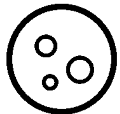
Callisto
