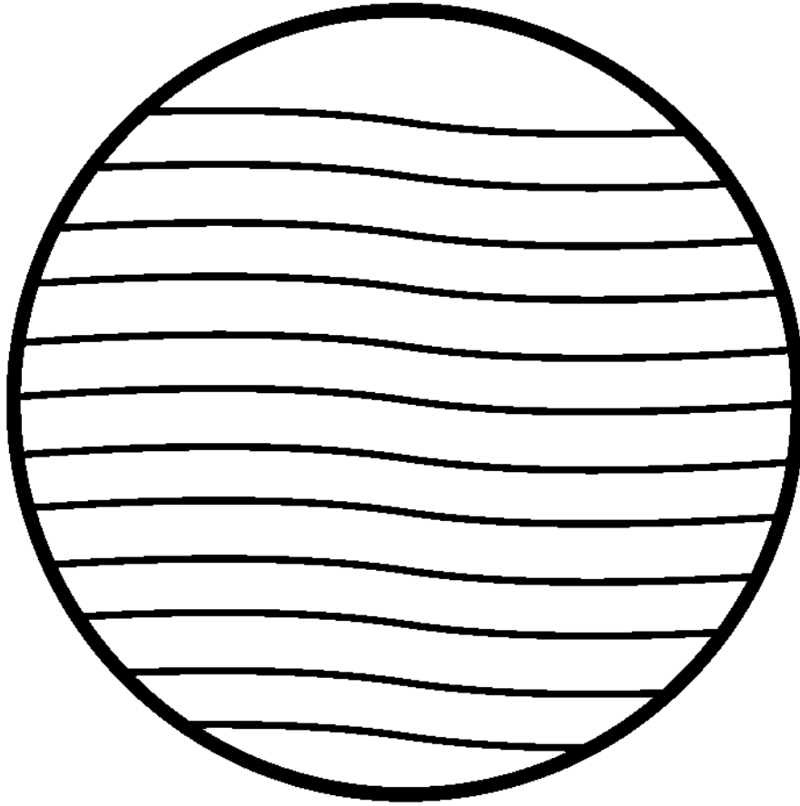
JUPITER
